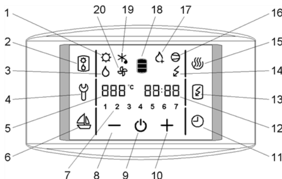
Bild 9: Bedienungsdisplay
